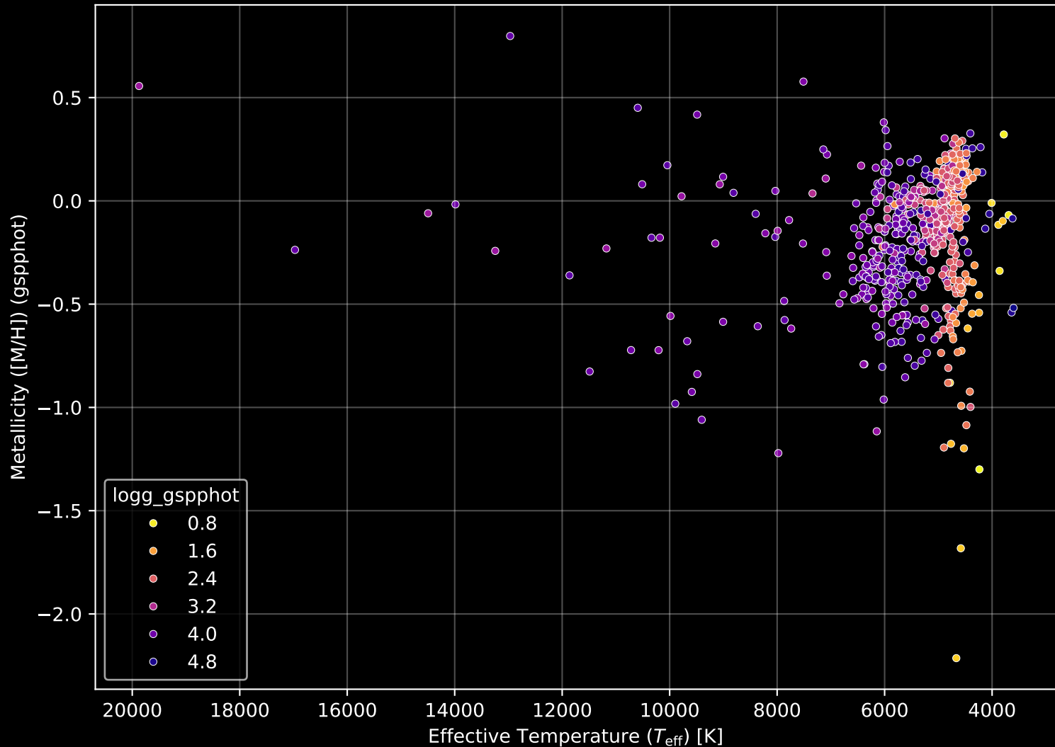
APOGEE DR17 Field: [K14_080+08] Stellar Population Parameters (n= 704)
